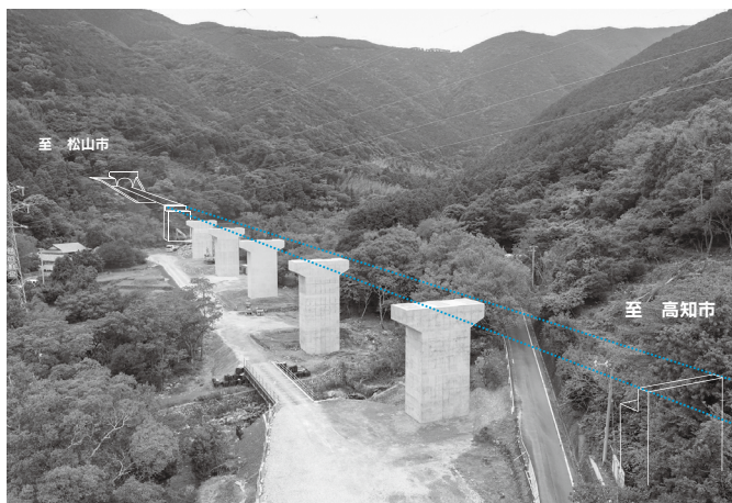
津島道路柏川橋（仮称）工事状況（愛南町柏地区）
